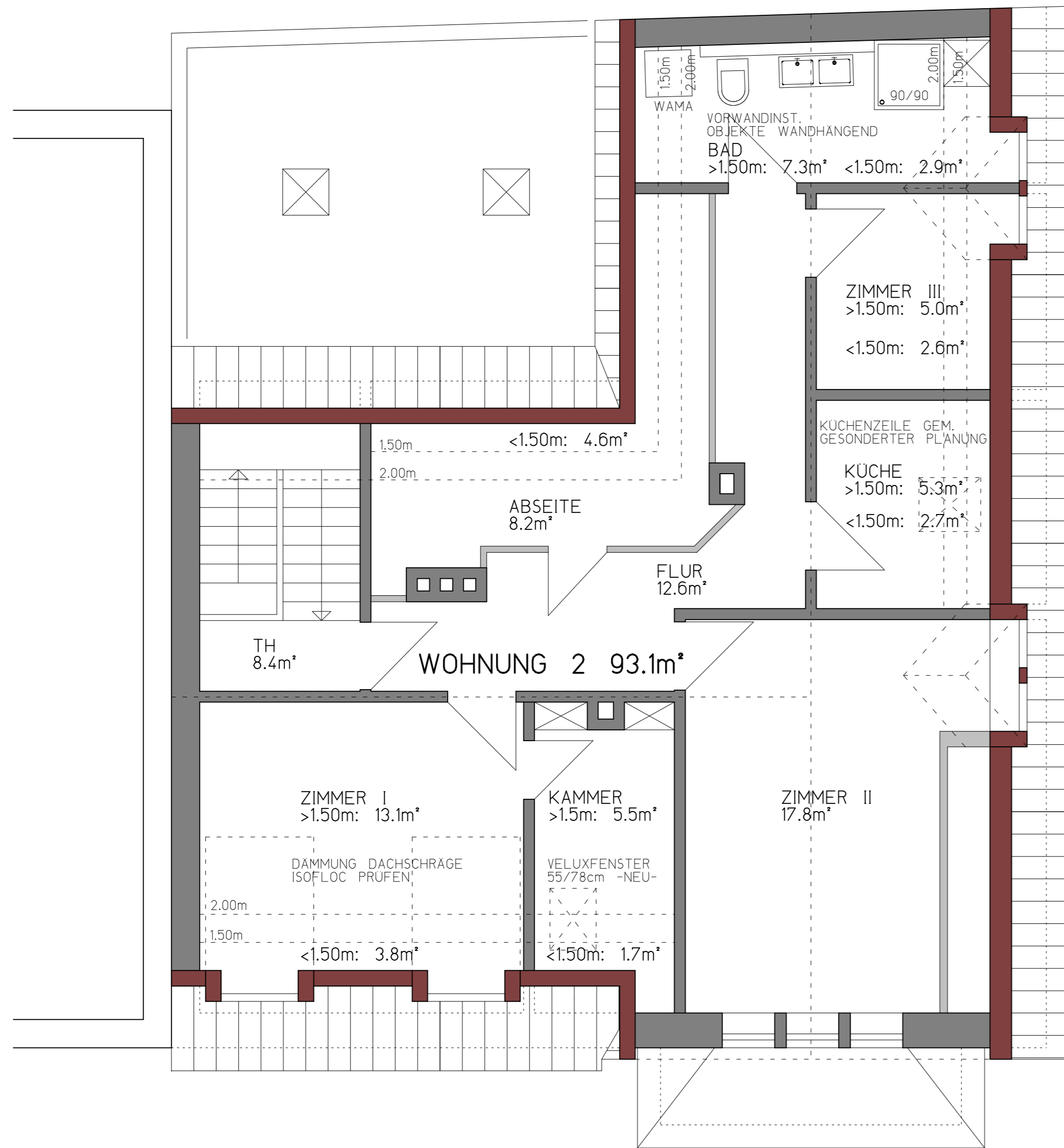
DACHGESCHOSS M 1:50
