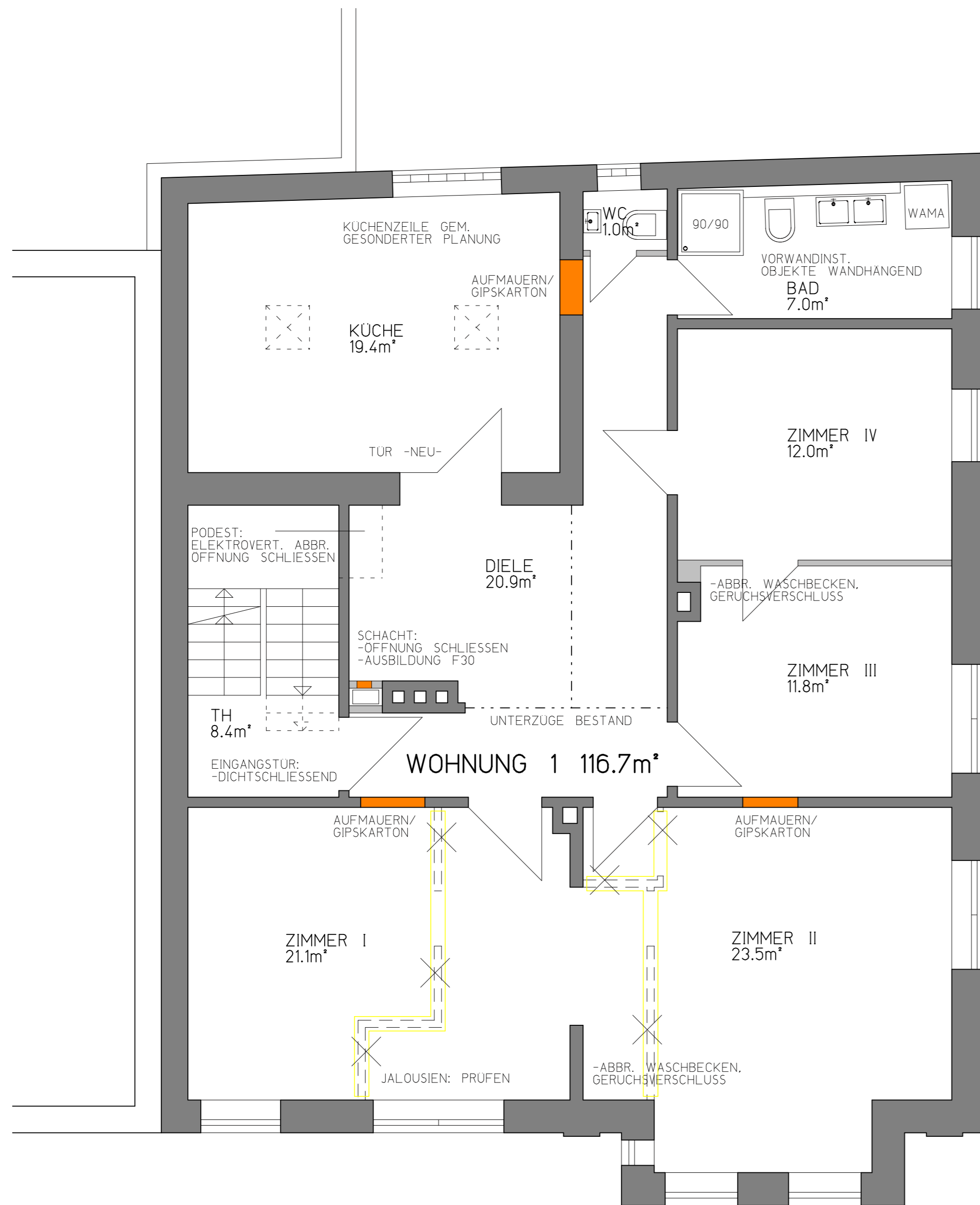
OBERGESCHOSS M 1:50
